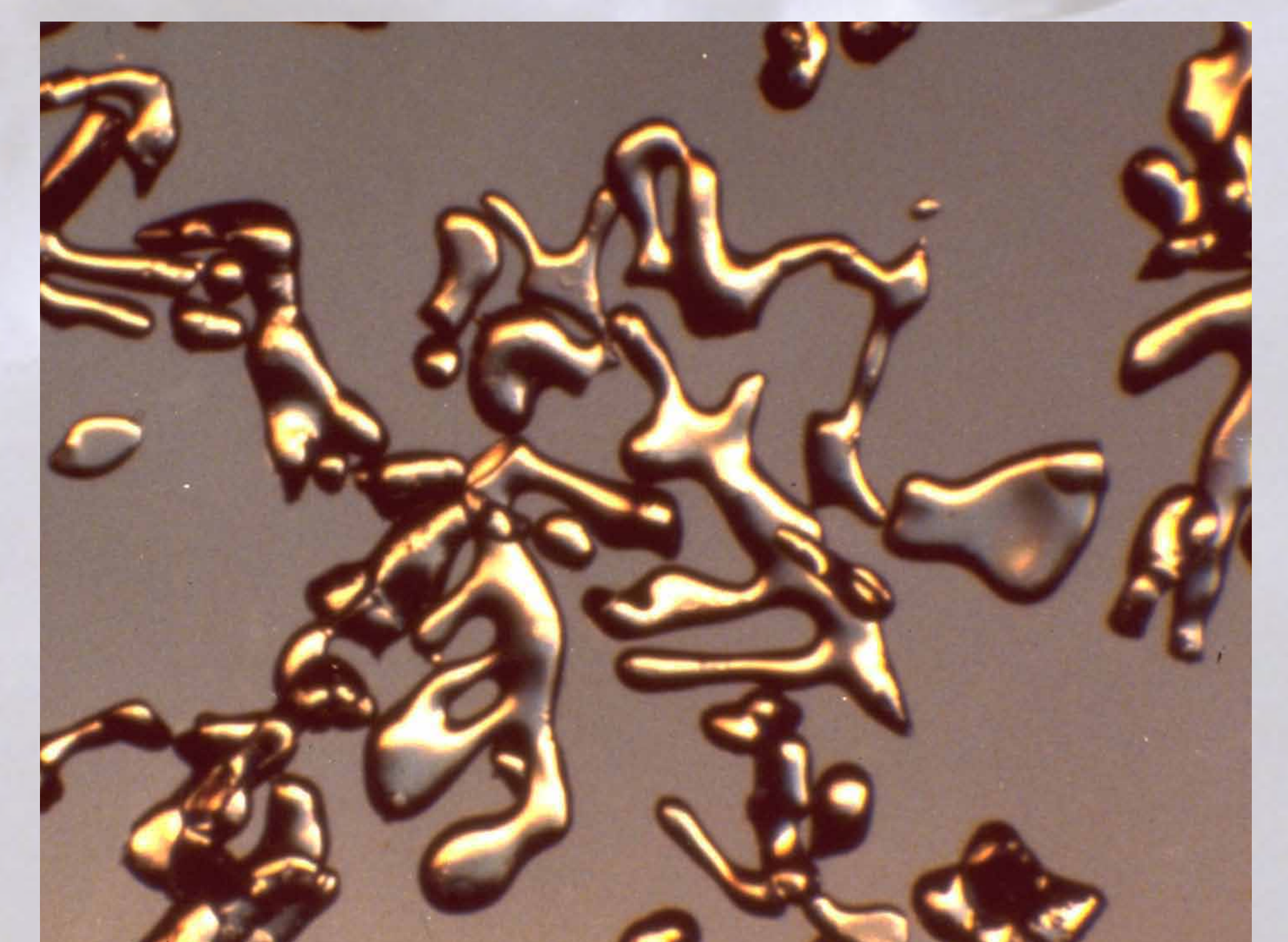
Cristaux ronds
